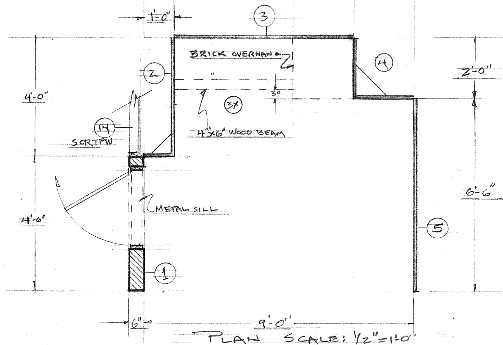
PLAN SCALE: 1/2" = 1'-0"
