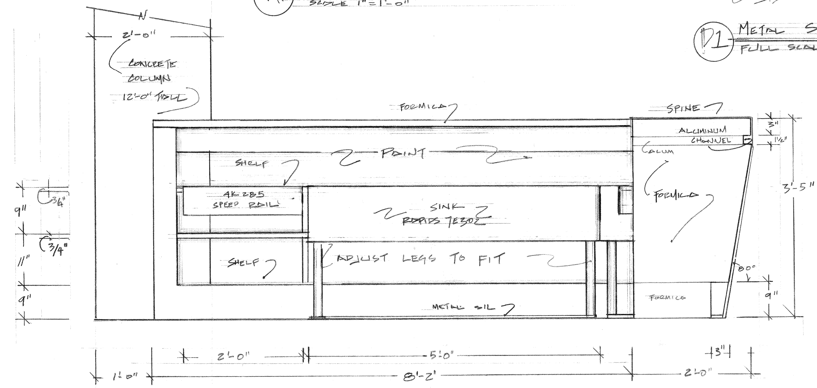
C U.S. BAR P/F SCALE 1"=1'-0"
