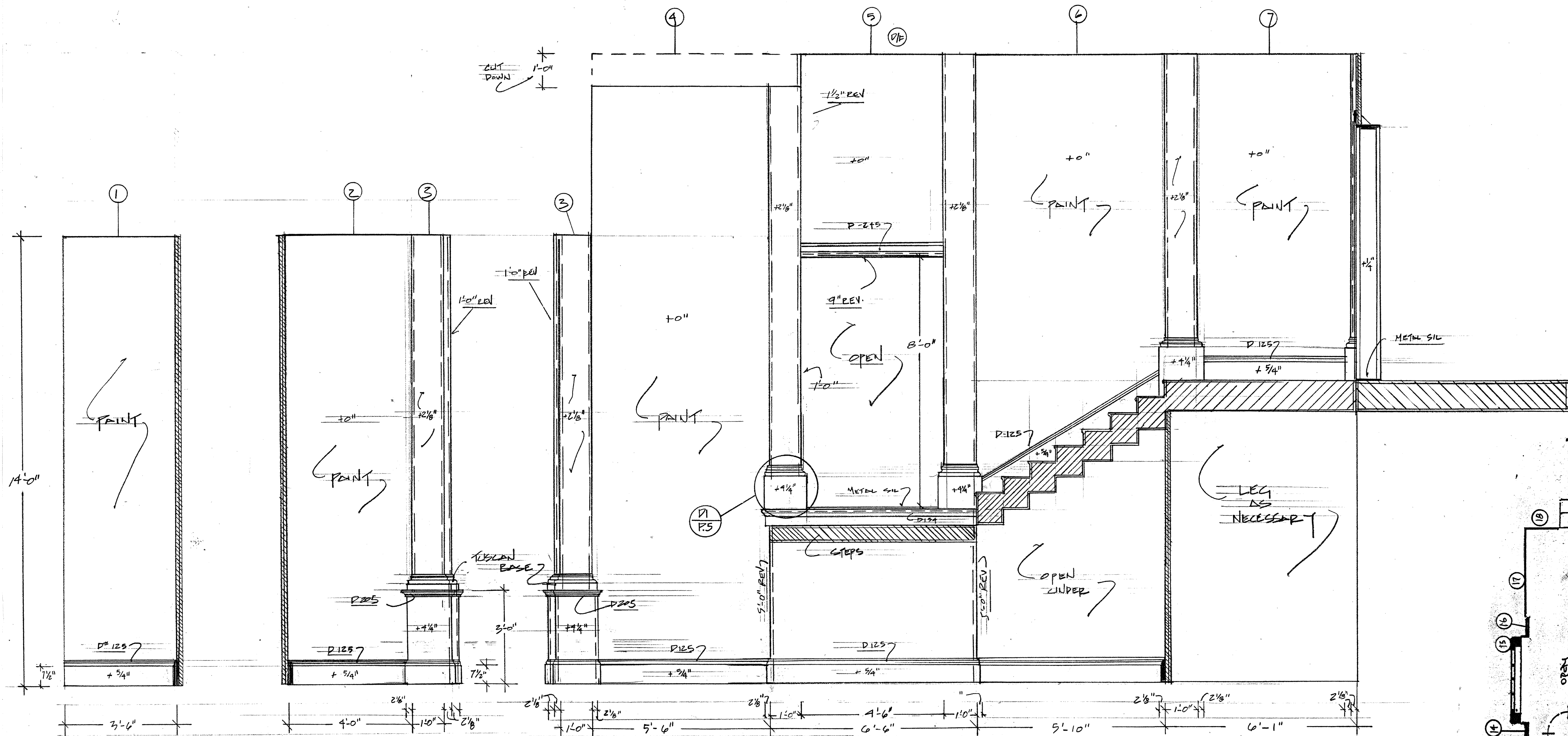
E. D. S. RIGHT WINGS SCALE 1/2" = 1'-0"
