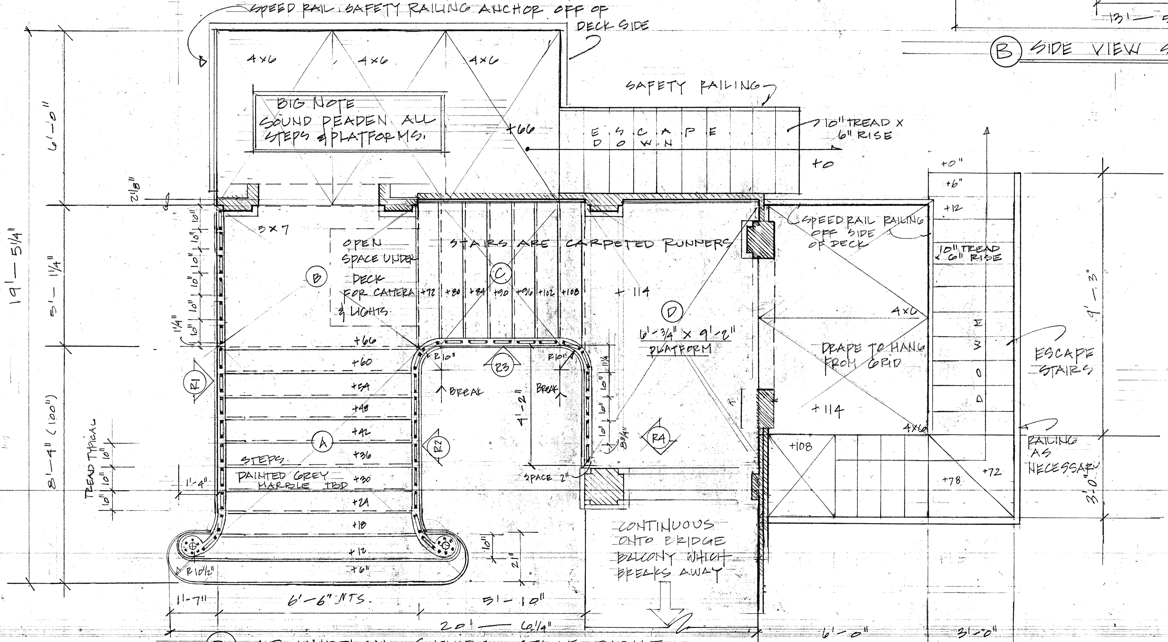
(D) GROUNDPLAN STAIRS STAGE RIGHT
