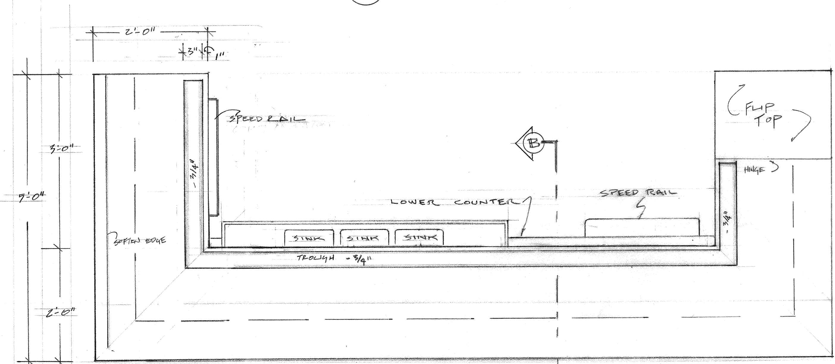
K BAR TOP SCALE: 1"=1'-0"
